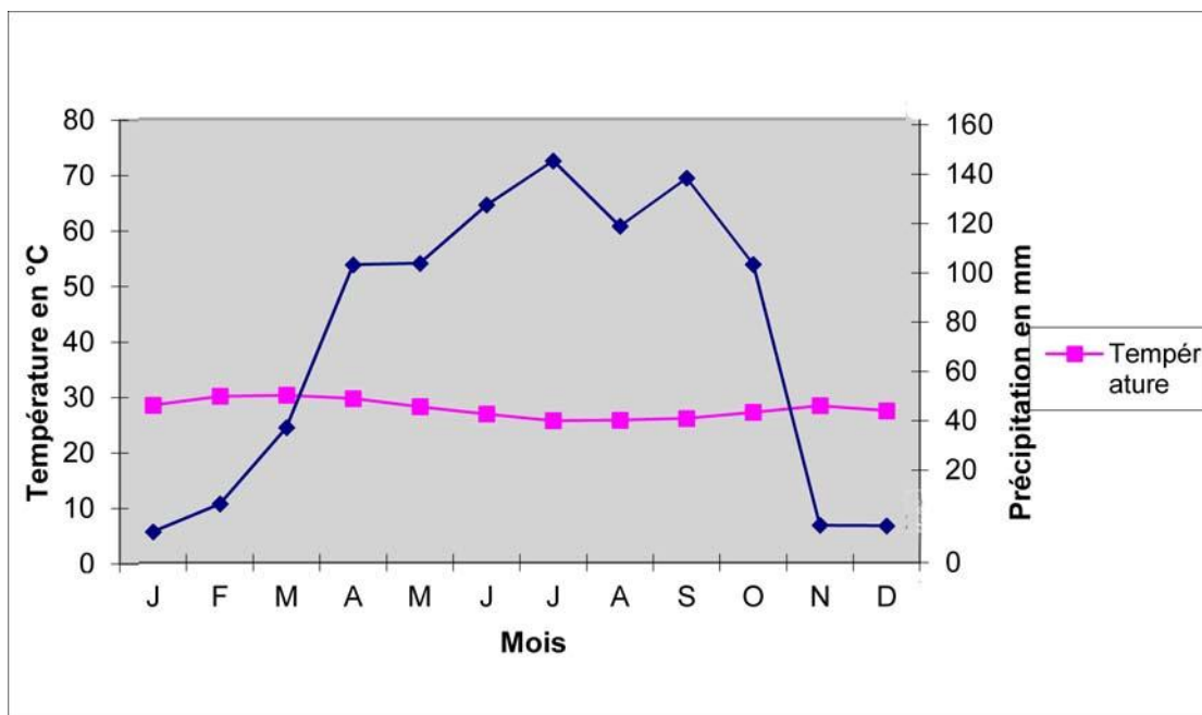
Figure 3 : Diagramme ombro-thermique : station de Ouèssè
